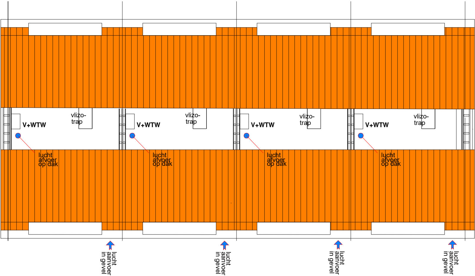
bergzoder - techniekruimte V+WTW= ventilatie met warmte terugwinning
